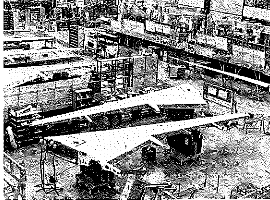
Planta de Aernnova de fabricación de aerestructuras.
